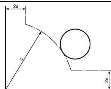
Расстояние от угла листа стекла до кромки отверстия
