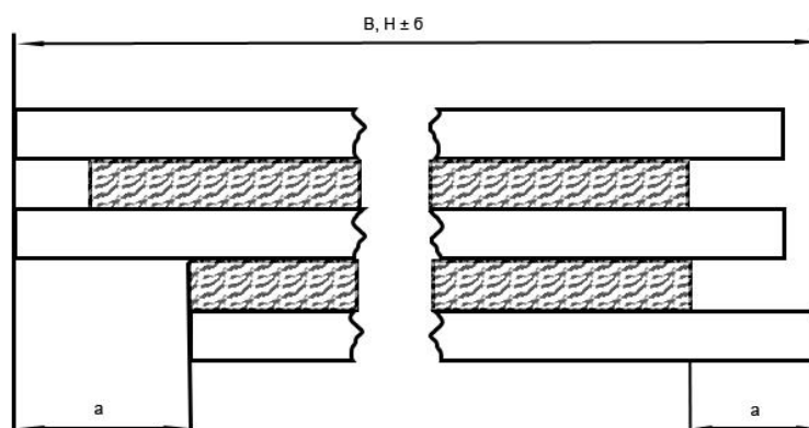
B, H – длина и ширина многослойного стекла. a – смещение листов стекла в многослойном стекле; b – допуск на длину и ширину многослойного стекла
