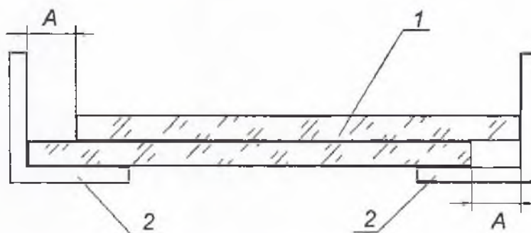
1 – контролируемое изделие (многослойное стекло, стеклопакет); 2 – угольник; А – смещение стекол
