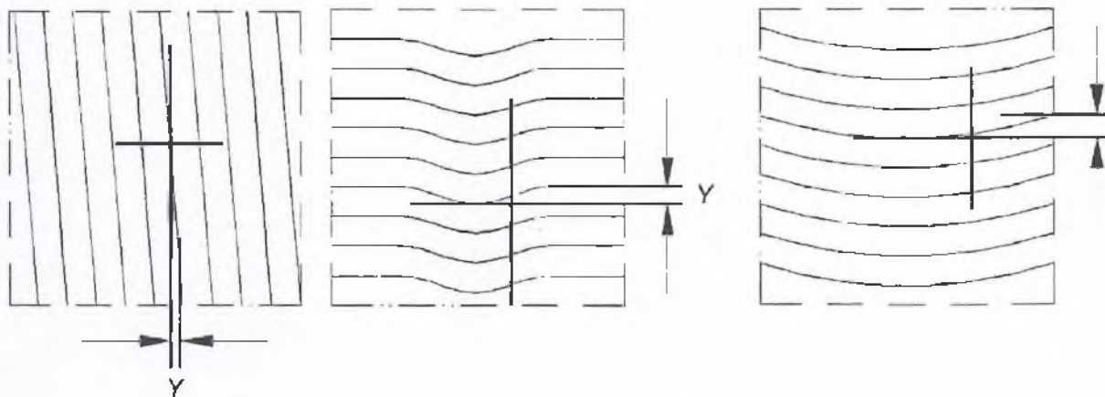
Y – смещение проволоки Рисунок 6 – Примеры смещения проволоки
